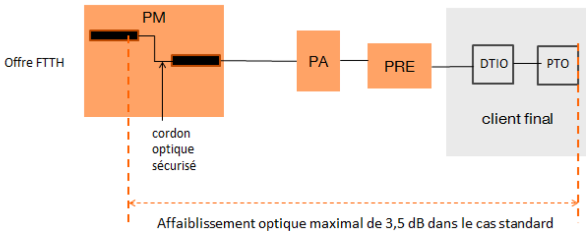
Figure 8 : FTTE passif au PM – affaiblissement maximal dans un cas standard
