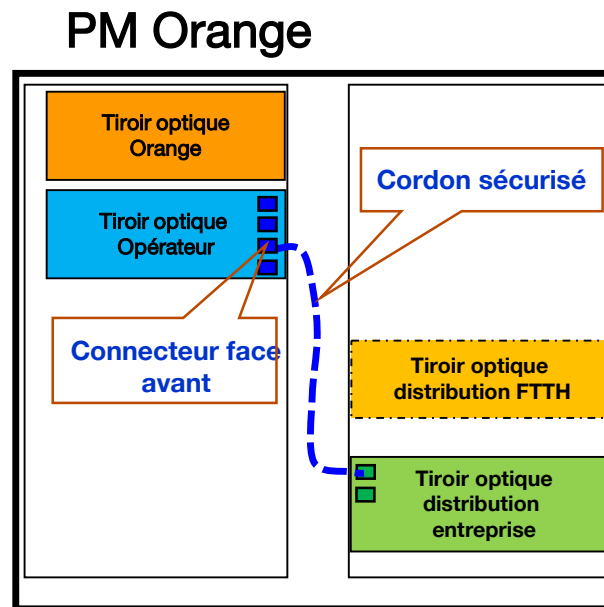
Figure 2 : FTTE passif au PM - Raccordement au PM
